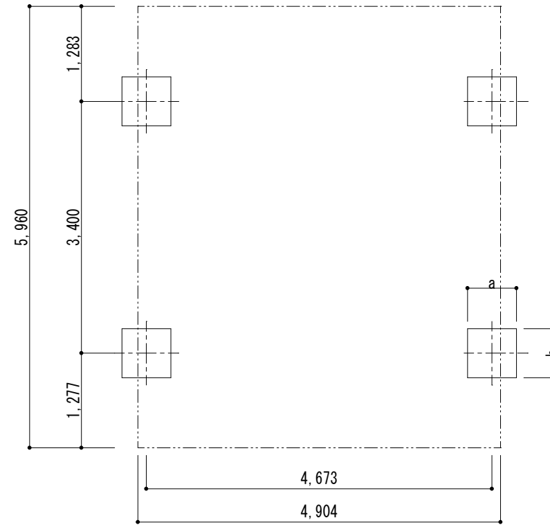
■ 基礎配置図
